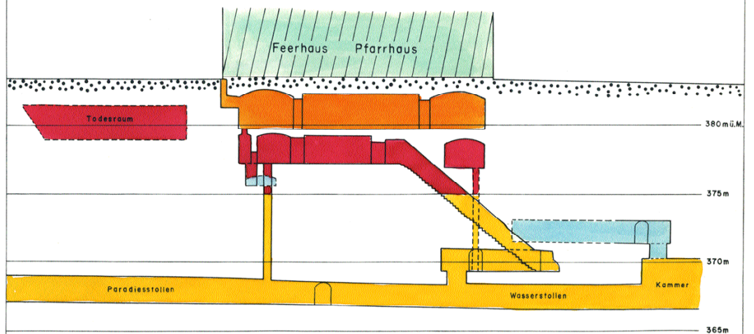
Längensprofil in süd-nördlicher Richtung 1:250
